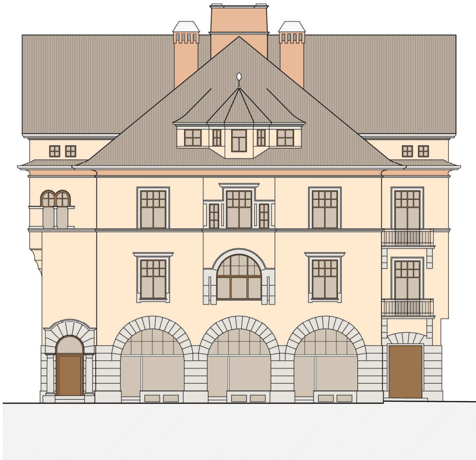
5.2 Ansicht Westen M=1:200
