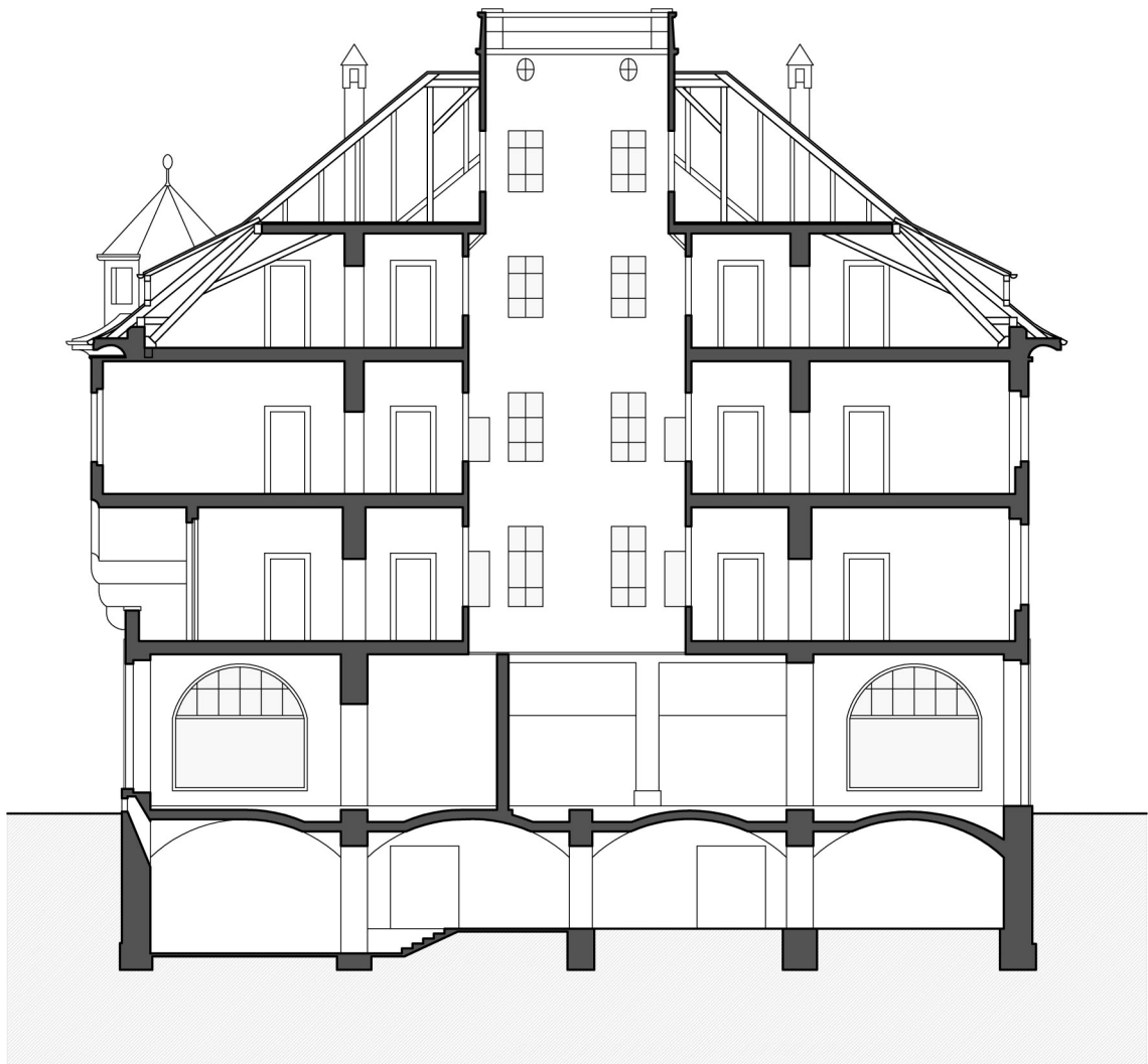
5.10 Schnitt A-A M=1:200
