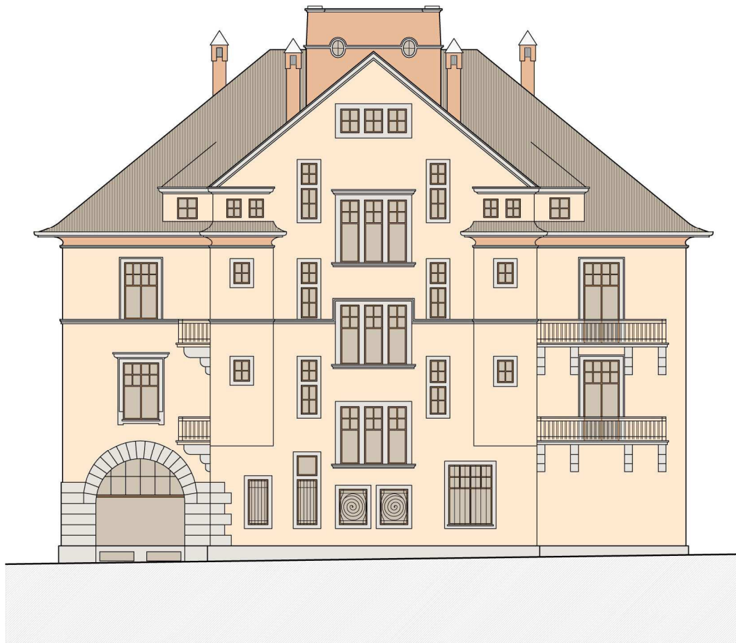
5.3 Ansicht Süden M=1:200
