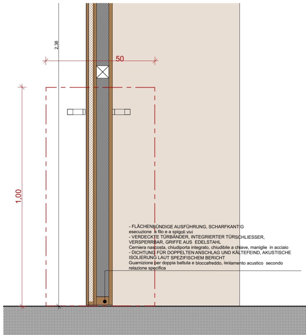
TÜRSCHNITT 1:10 sezione porta 1:10
