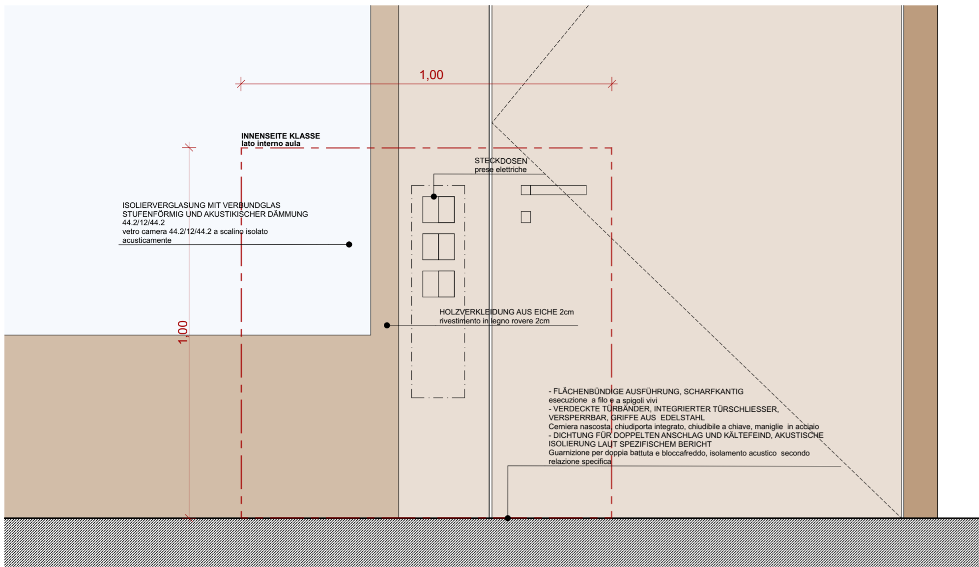
INNENANSICHT KLASSE 1:10 vista interna 1:10
