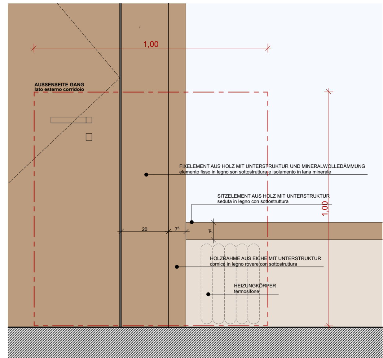
SITZELEMENT SCHNITT 1:10 sezione seduta 1:10
