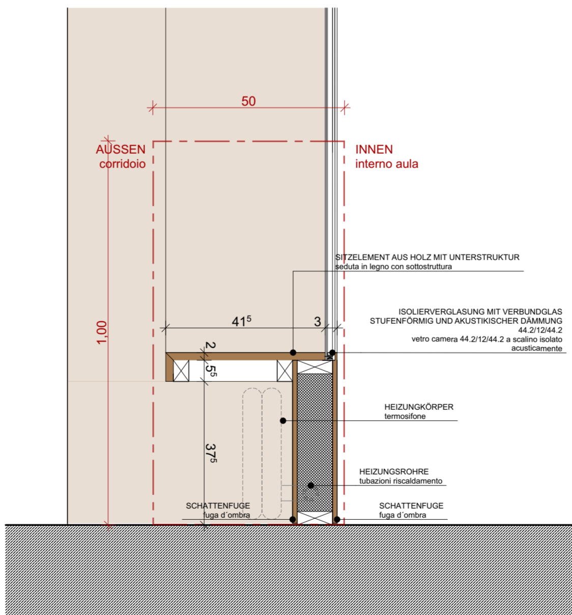
SITZELEMENT SCHNITT 1:10 sezione seduta 1:10
