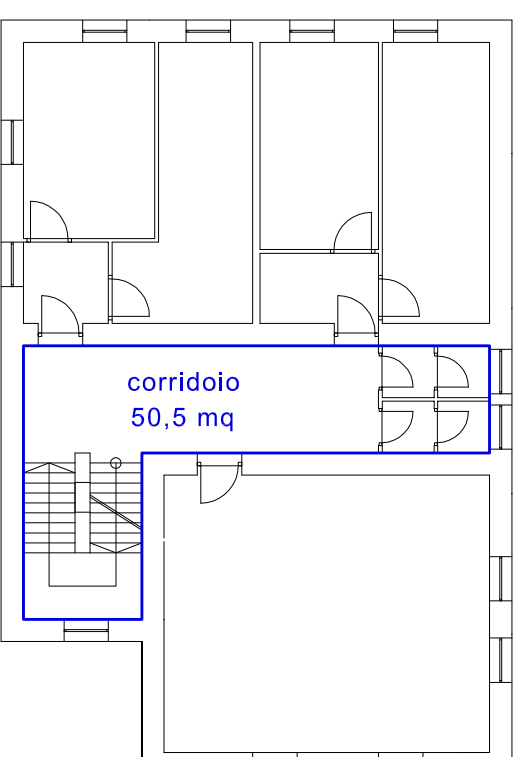
PIANO PRIMO
