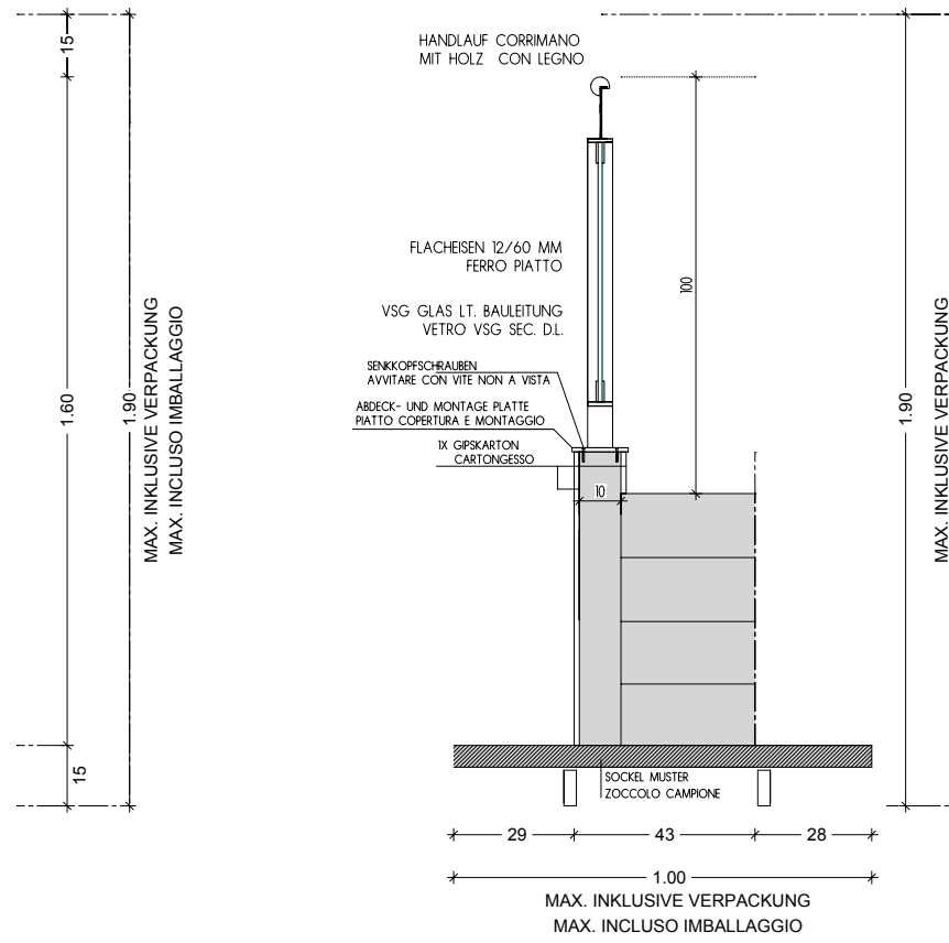
SCHNITT SEZIONE
