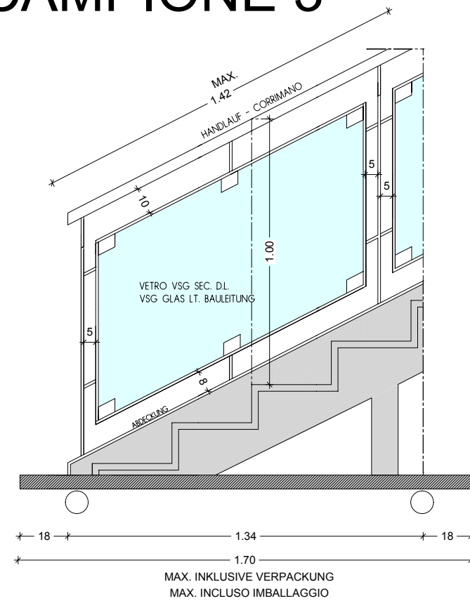
ANSICHT FACCIATA
