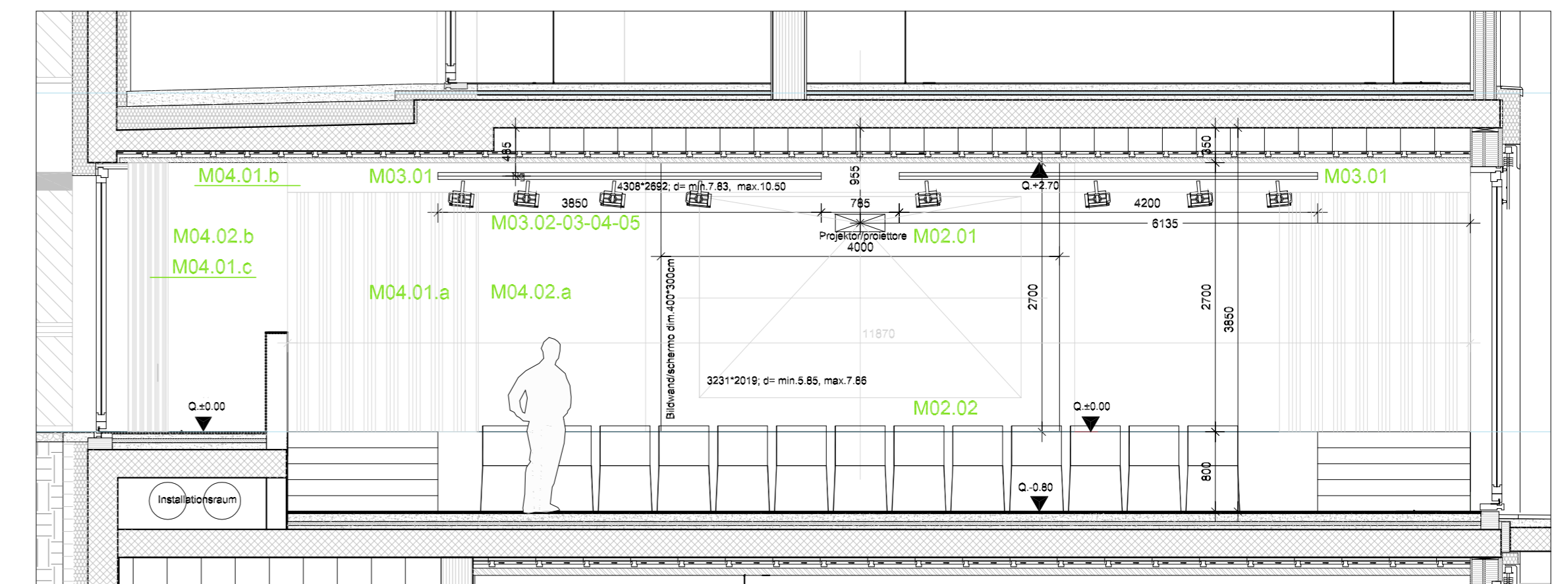
SCHNITT B-B / SEZIONE B-B 1:50
