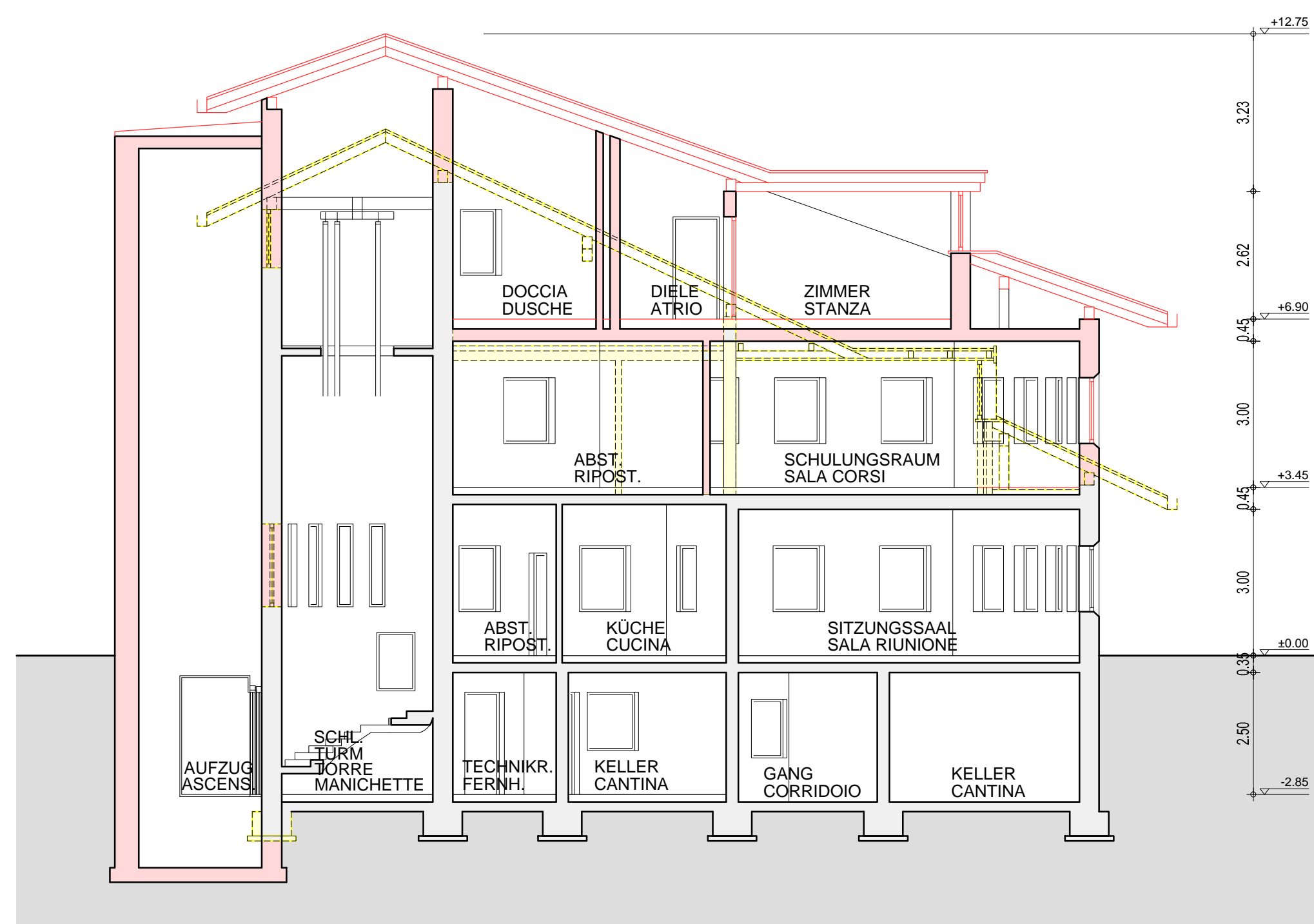
SCHNITT A-A - SEZIONE A-A 1:100
