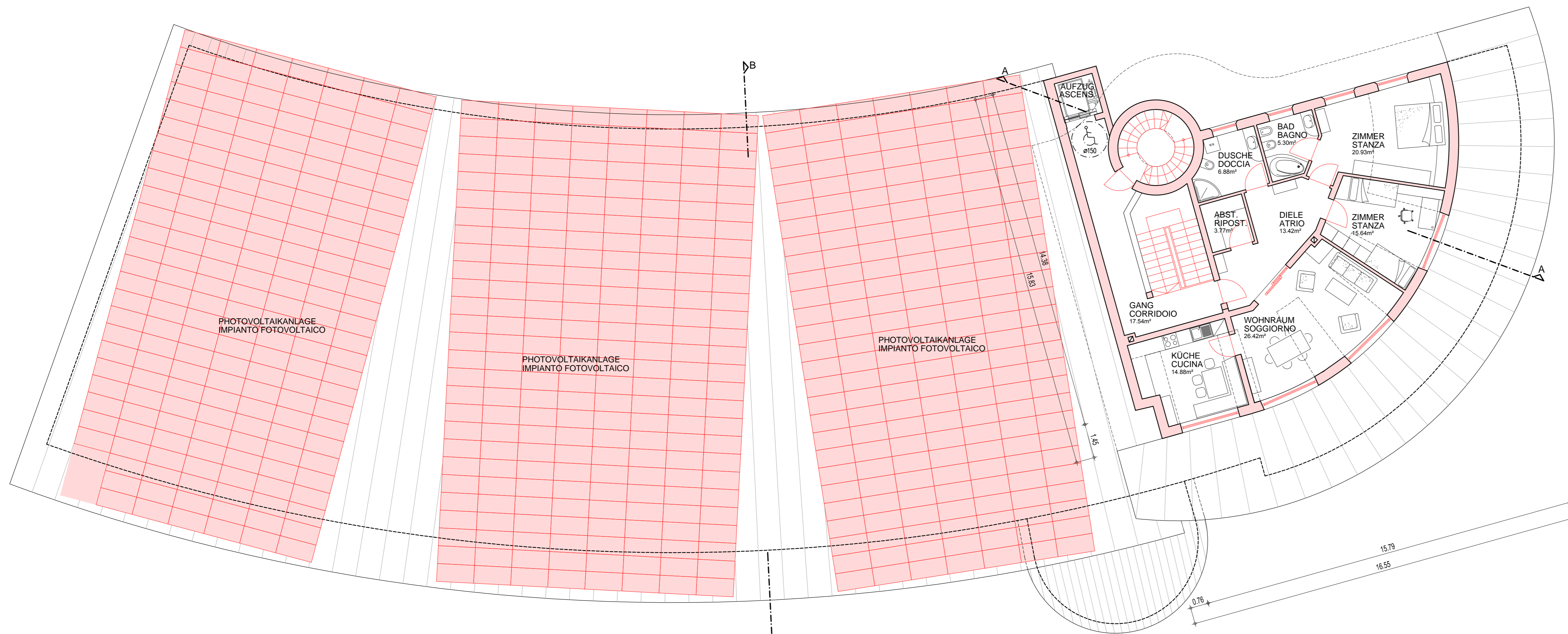
DACHGESCHOSS - SOTTOTETTO 1:100
