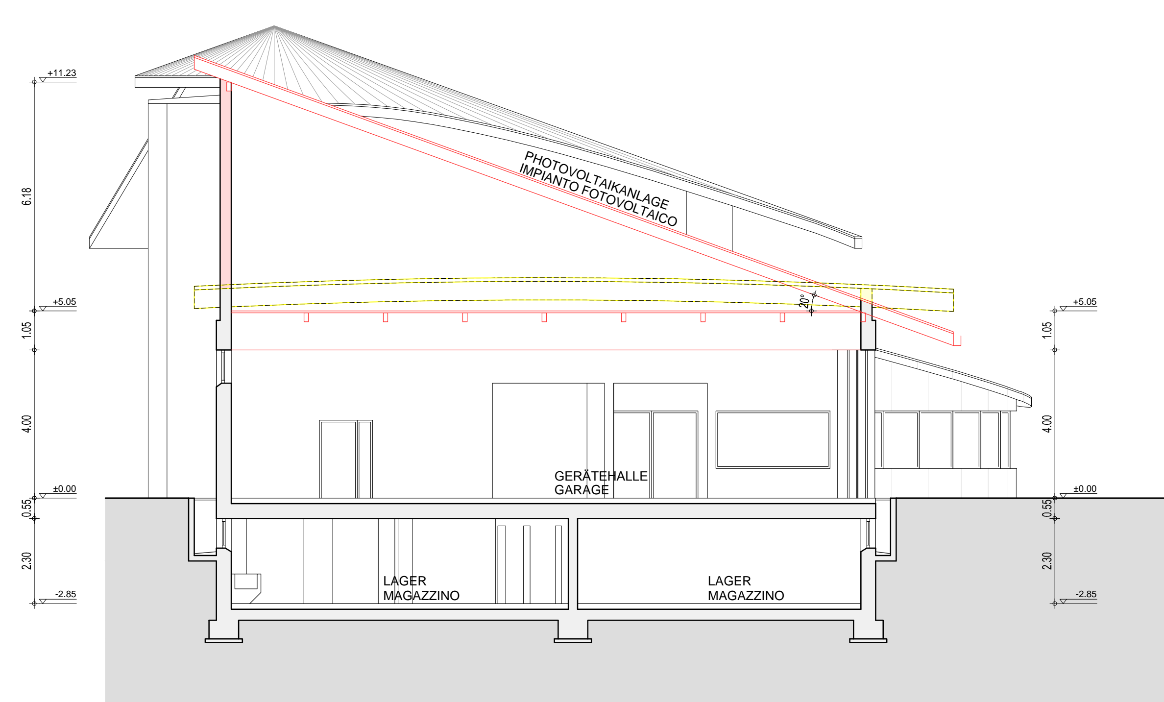
SCHNITT B-B - SEZIONE B-B 1:100
